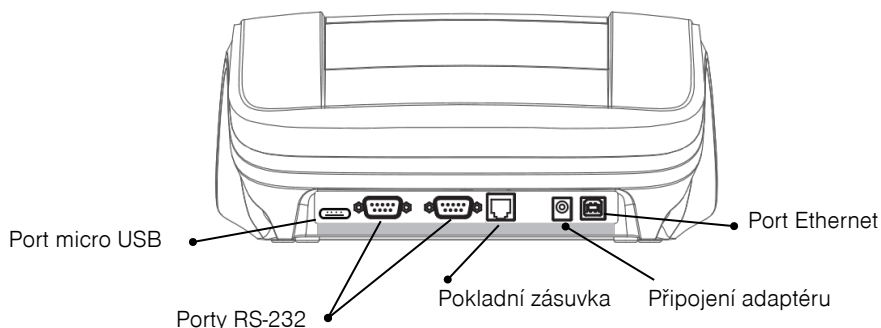
Obrázek 2.2 – Konektory pokladny Euro-150TEi Flexy CZ
